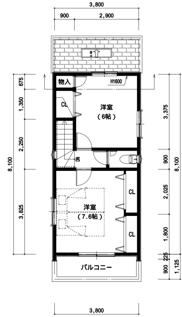
3階 平面図
