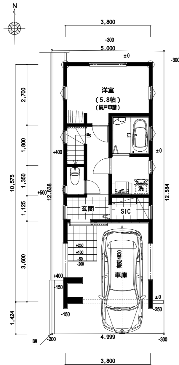
1階 平面図
