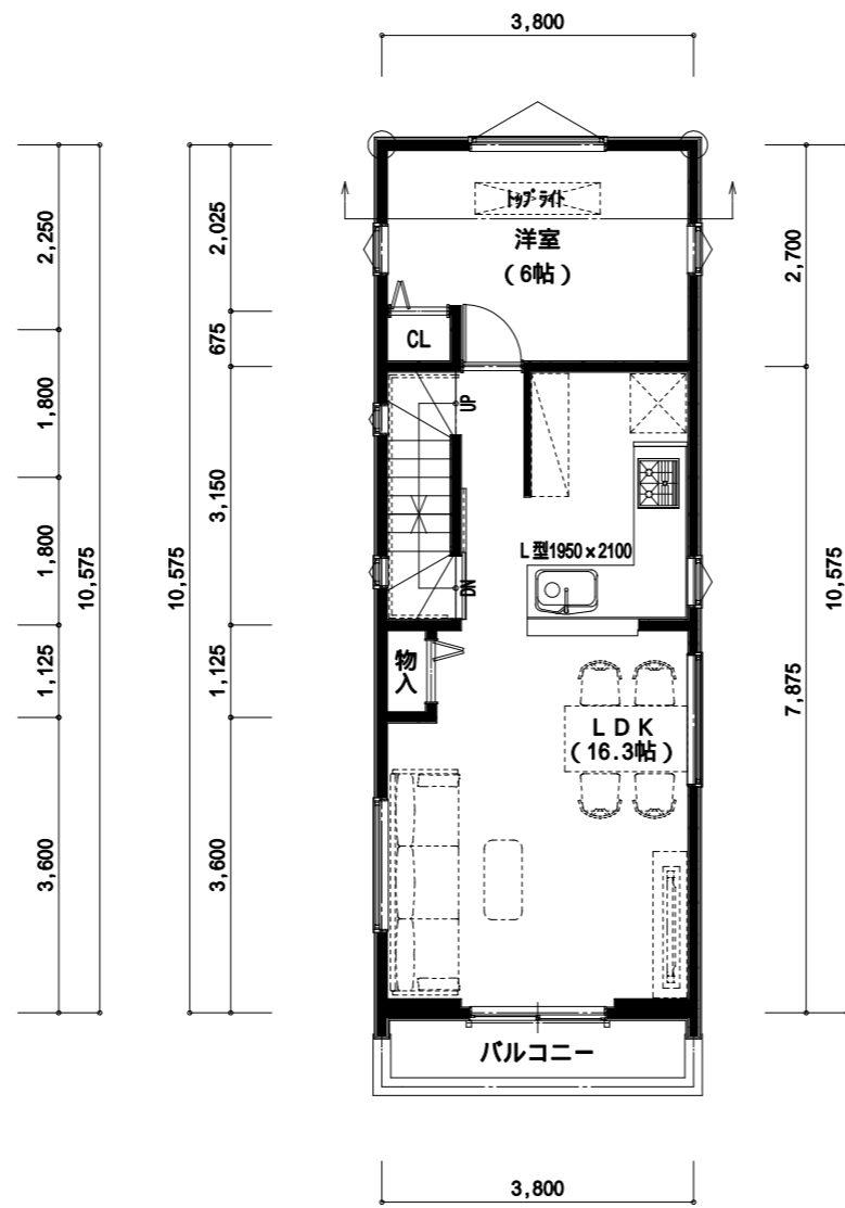
2階 平面図
